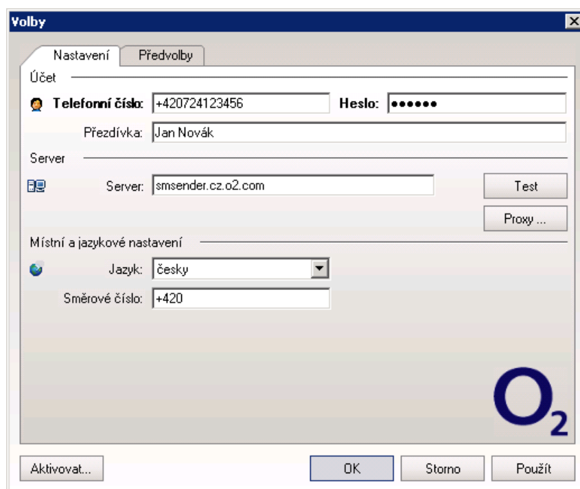
Obrázek 5 – Dialog „Možnosti“
