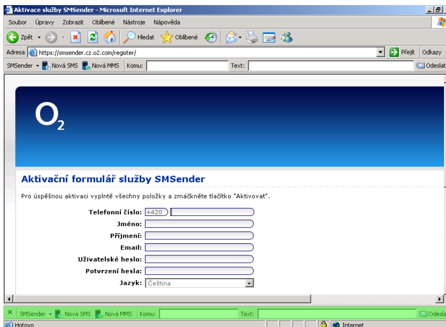
Obrázek 2 – Explorer Bar
